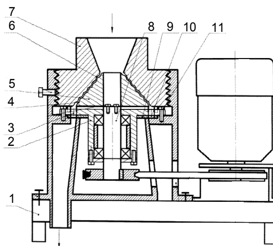
Рис. 7. Конусная инерционная дробилка: 1 – корпус; 2 – пластина-дозатор с технологическим отверстием; 3 – технологическое отверстие; 4 – правая навивка внутреннего конуса; 5 – внутренний конус; 6 – левая навивка наружного конуса; 7 – наружный конус; 8 – вал приводной; 9 – прокладка; 10 – технологическое отверстие; 11 – регулирующая пластина [24]
