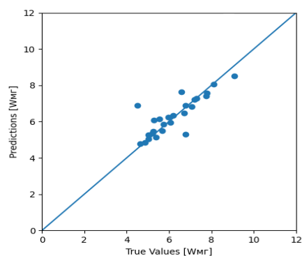
Рис. 3. Результаты прогнозирования функцией Linear параметра W_{mr}
